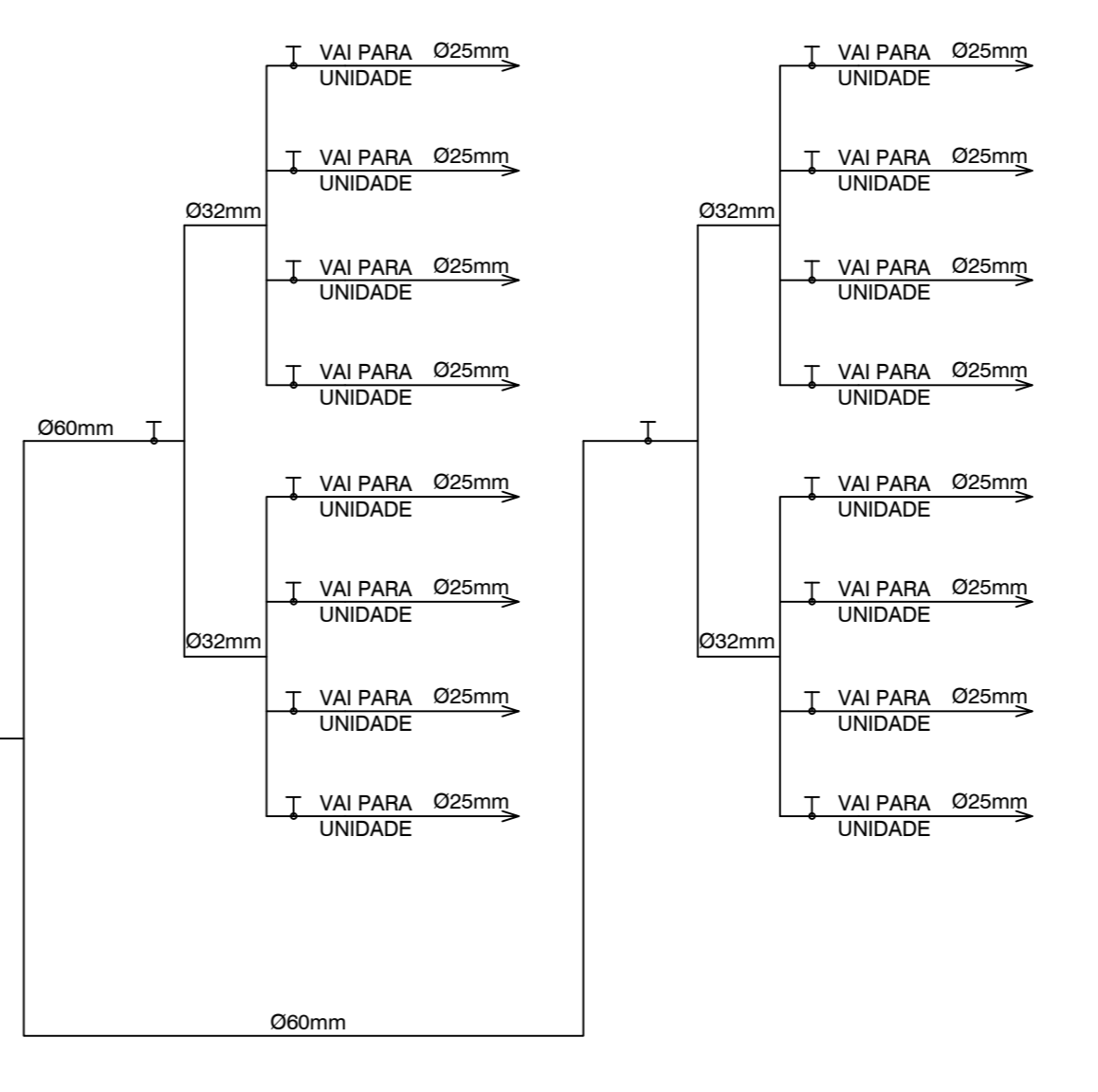
Esquema Vertical Reservatório e Distribuição ESC.: 1/75
