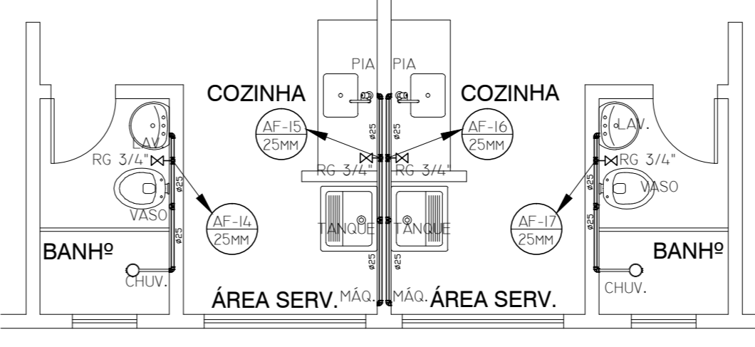
DETALHE TÉRREO ESC.: 1/50
