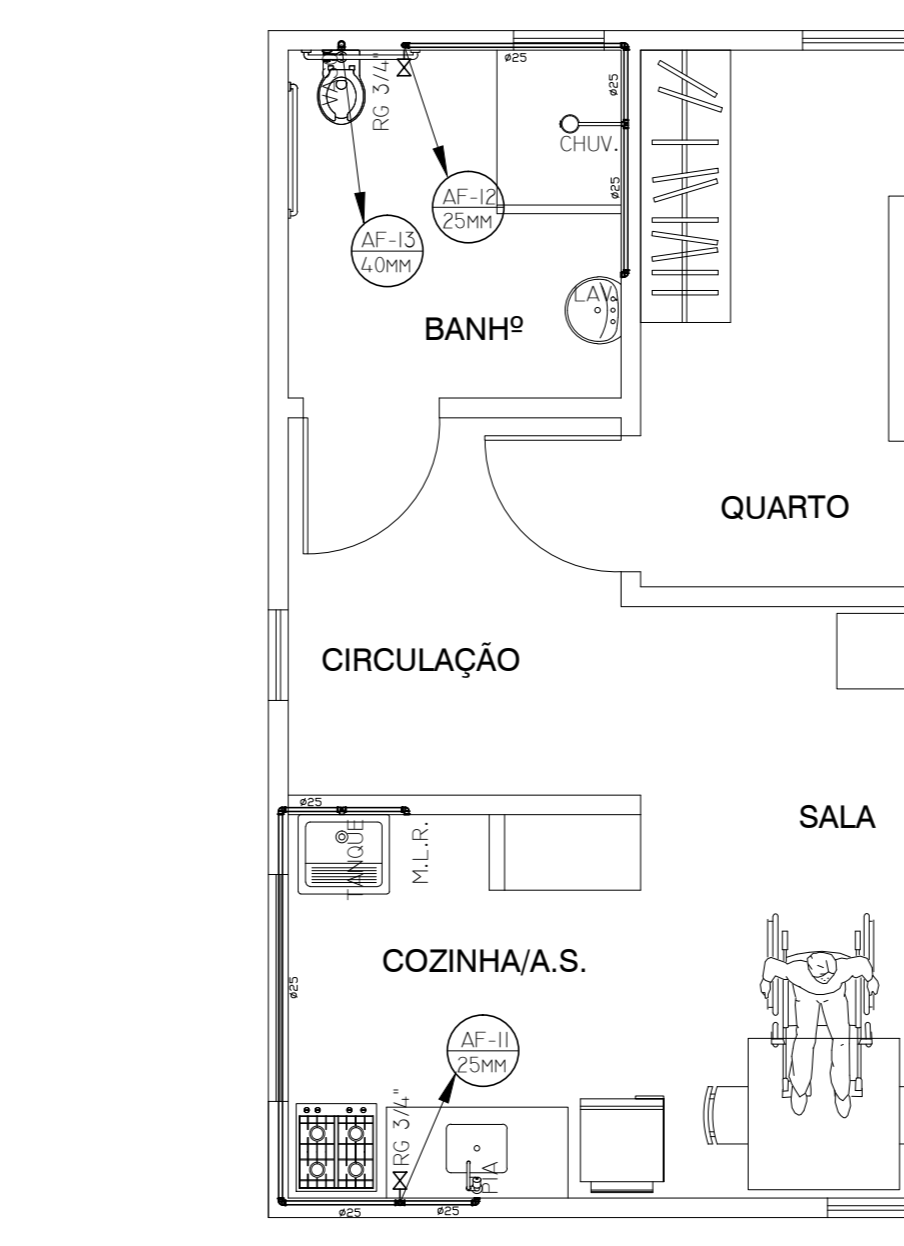
DETALHE TÉRREO ESC.: 1/50
