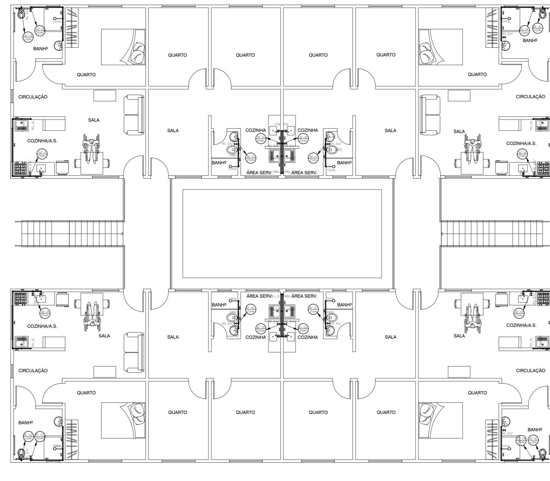
INSTALAÇÃO DE ÁGUA FRIA TÉRREO ESC.: 1/100
