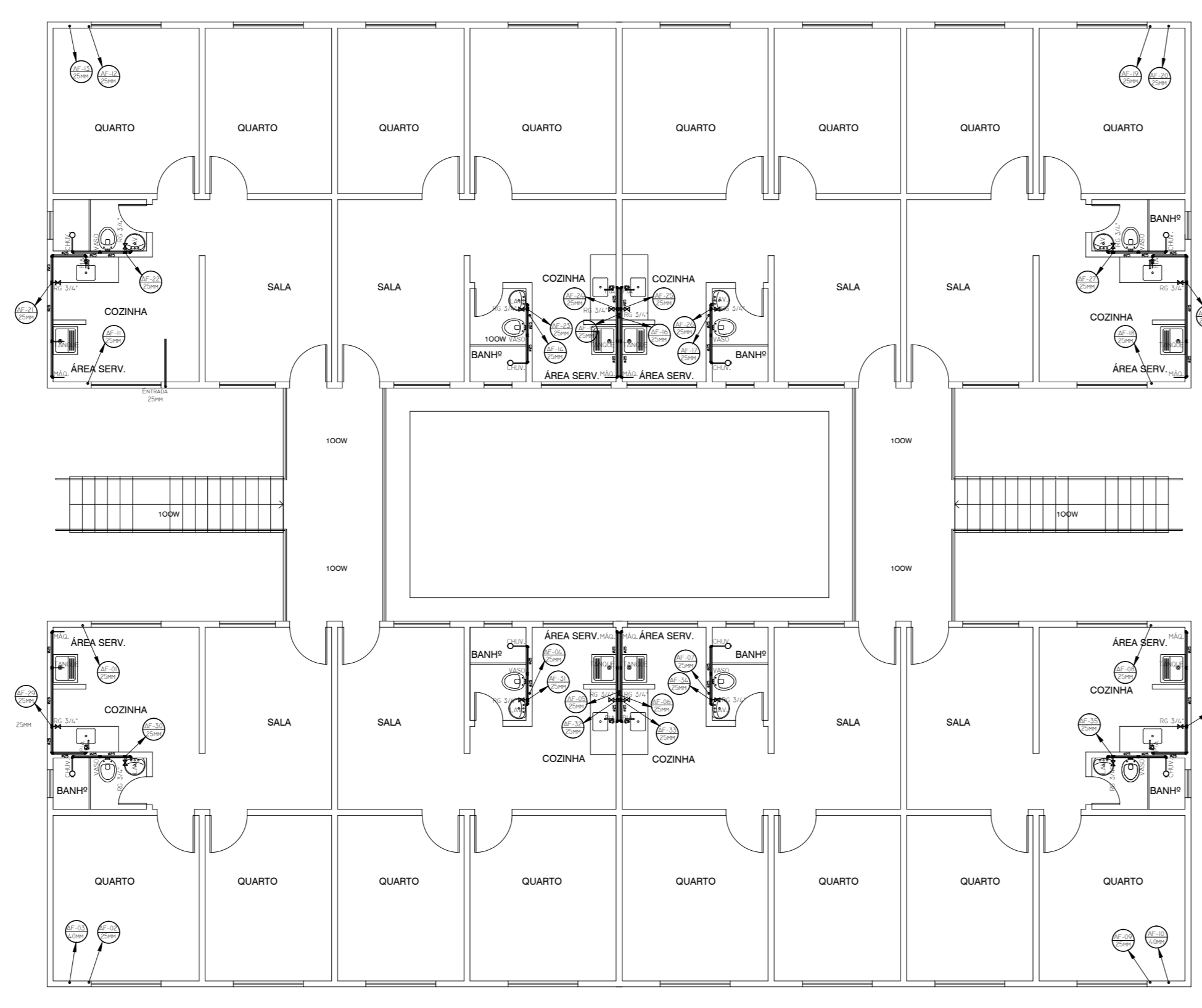
INSTALAÇÃO DE ÁGUA FRIA 1º PAV ESC.: 1/100
