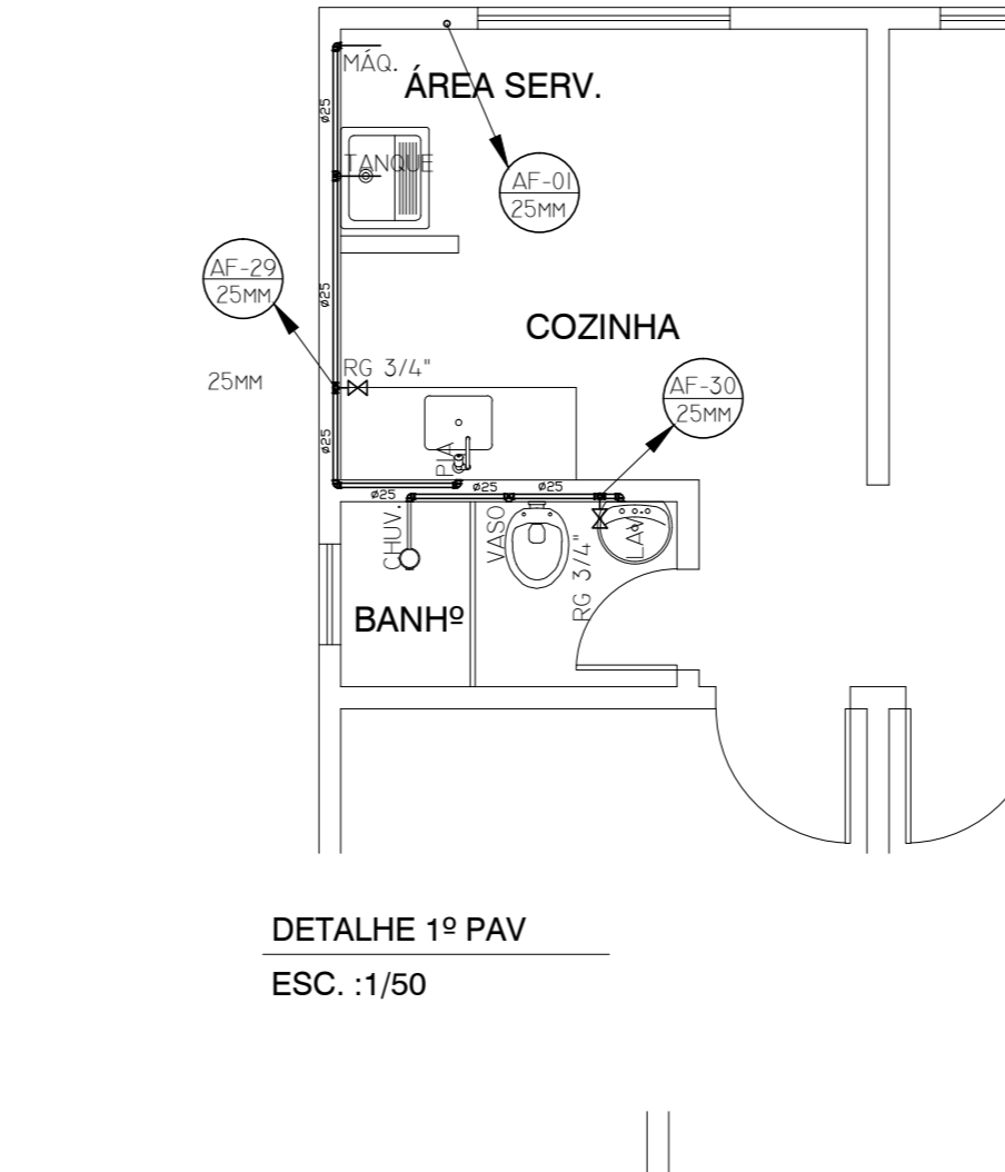
DETALHE 1º PAV ESC.: 1/50
