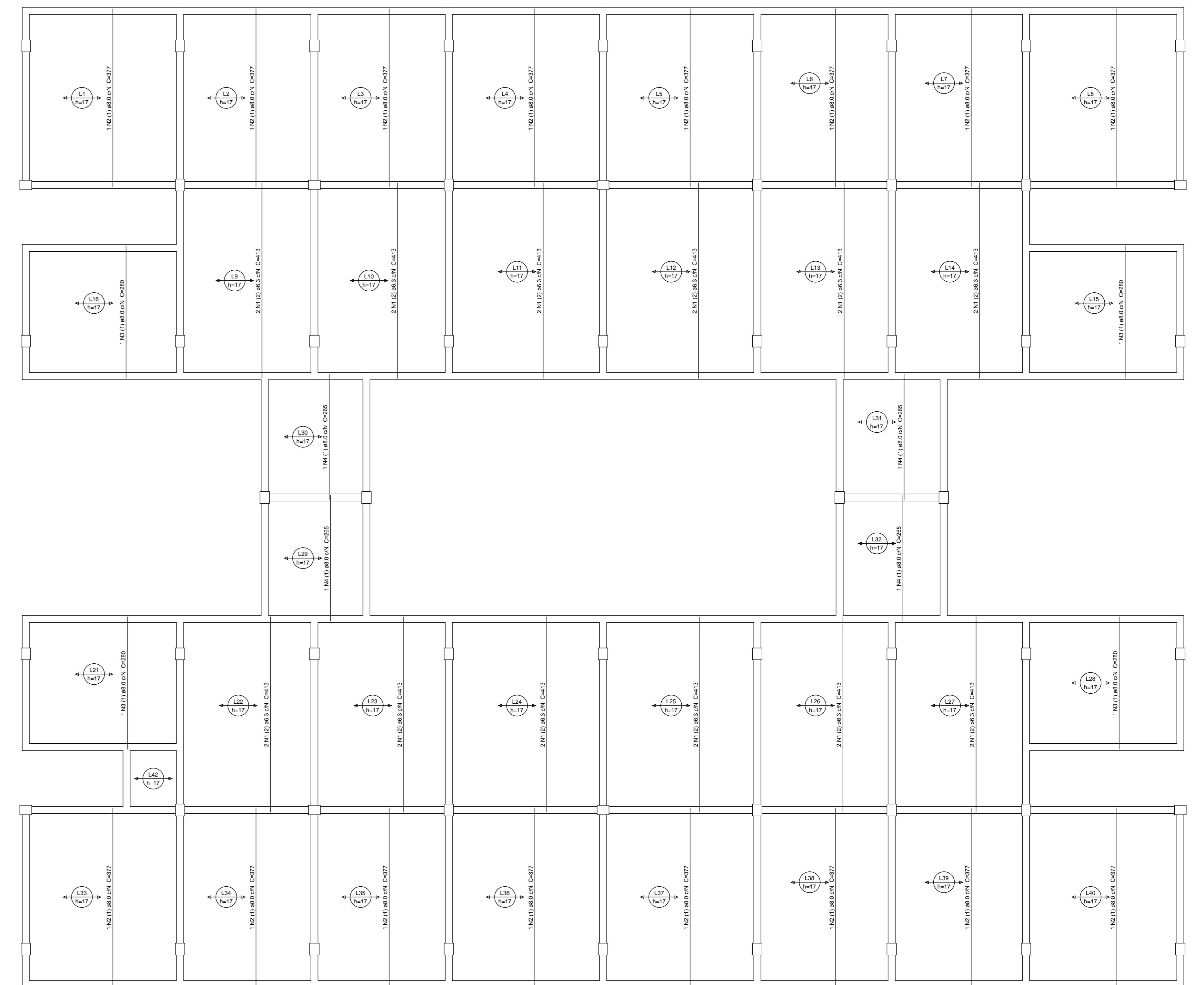
Armação posada das lajes do pavimento COB (lajes) ESCALA 1:50
